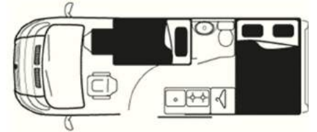
Vista 3 End Bed Night
