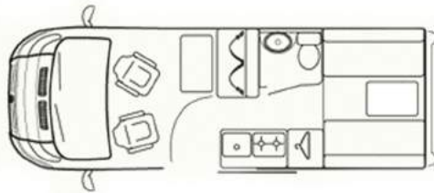
Vista 3 End Lounge Day
